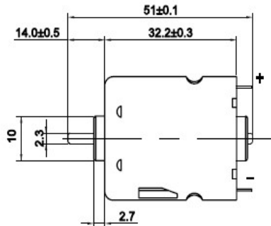
马达外形图 motor shape diagram
